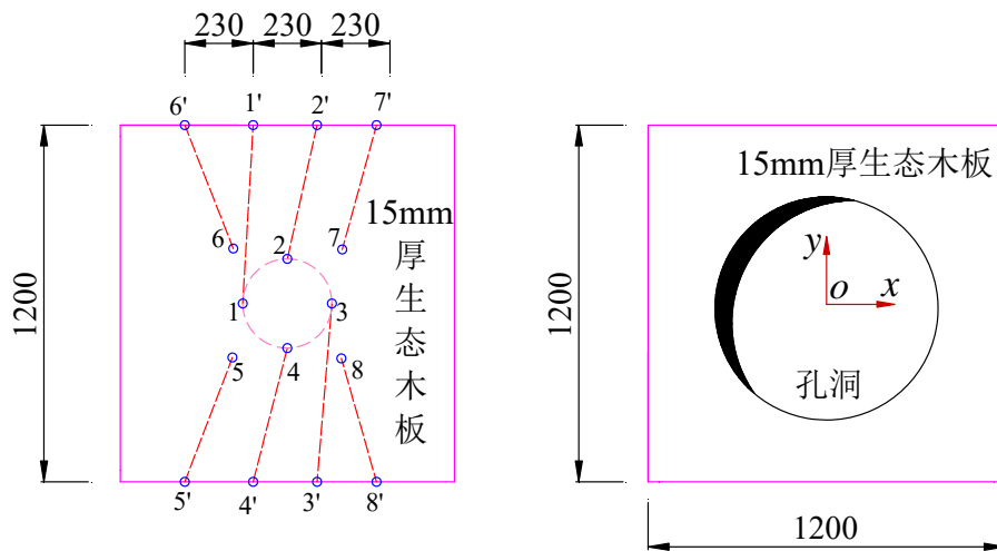
标高0.615m处平面图滑轮布置图
